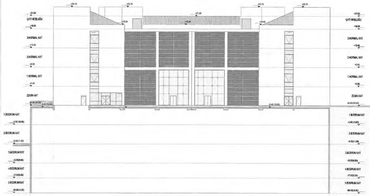
KUZAY CEPHESİ ÖLÇEK : 1/100
