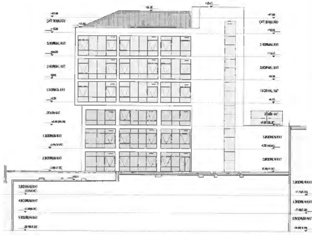
DOĞU CEPHESİ ÖLÇEK :1/100
