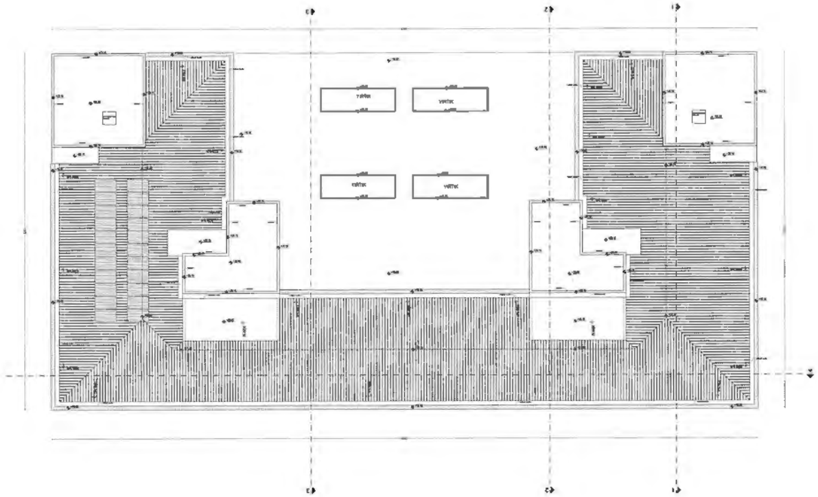
ÇATI BOŞLUĞU ÖLÇEK :1/100
